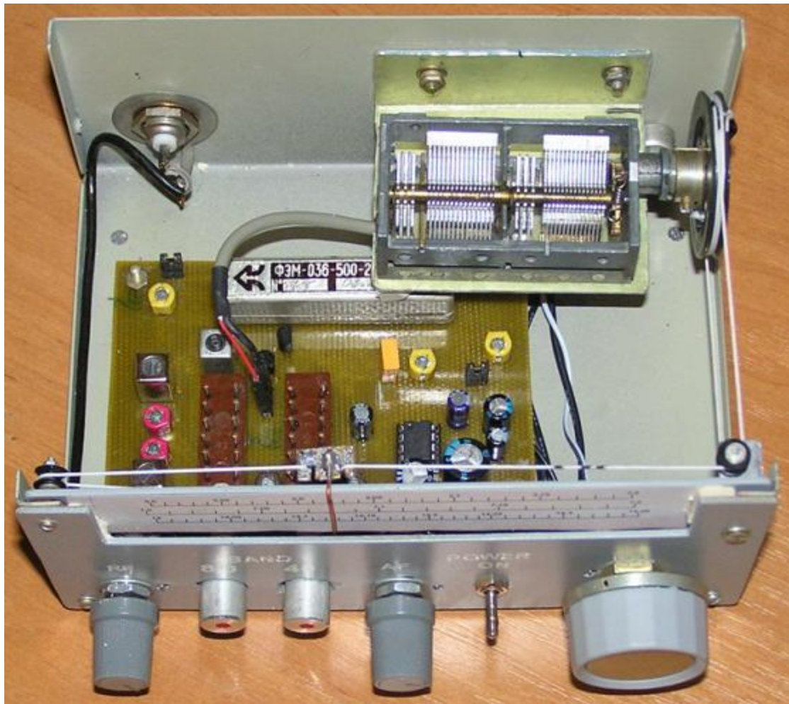
Рис. 2.9. Трехдиапазонный приёмник радиолобителя-наблюдателя на диапазоны 20, 40 и 80 м.
