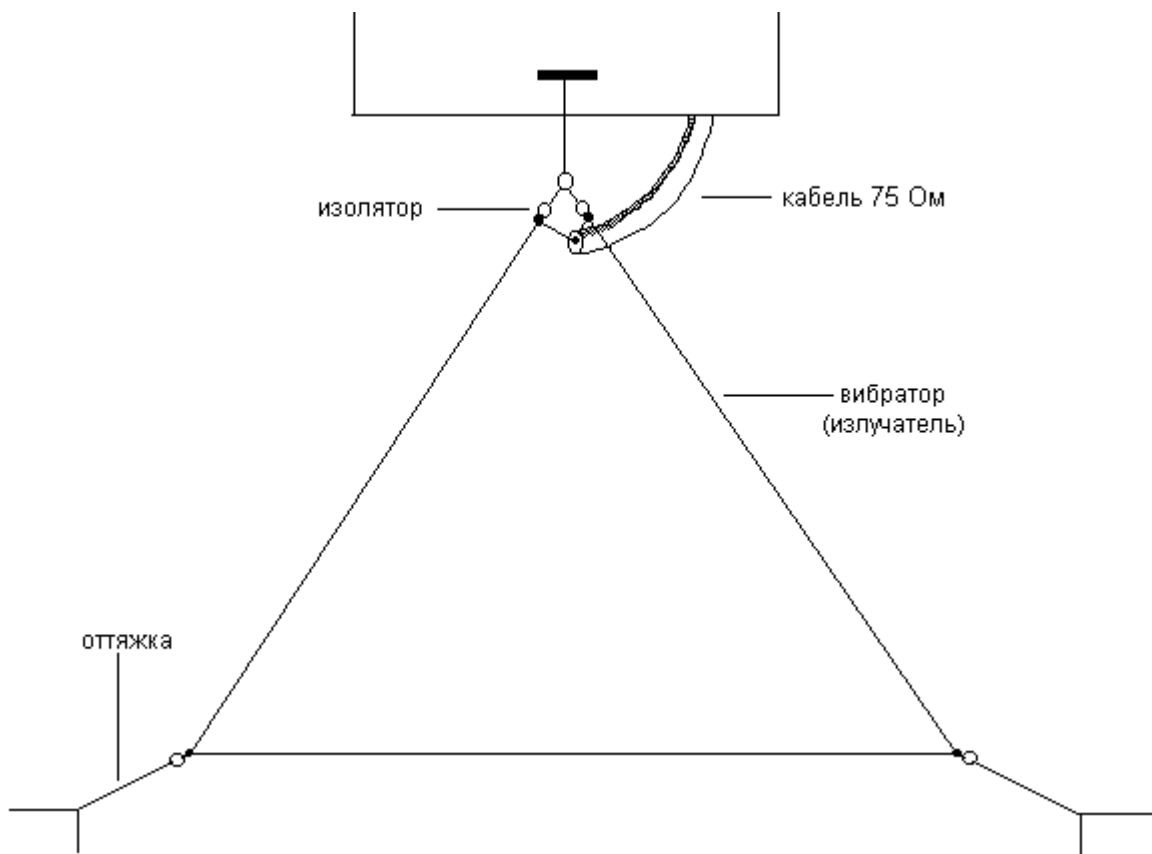
Рис. 2.15. Антенна «треугольник»
