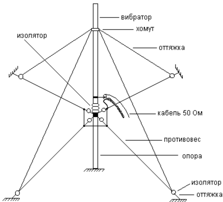
Рис. 2.16. Антенна «граунд-плэйн»
