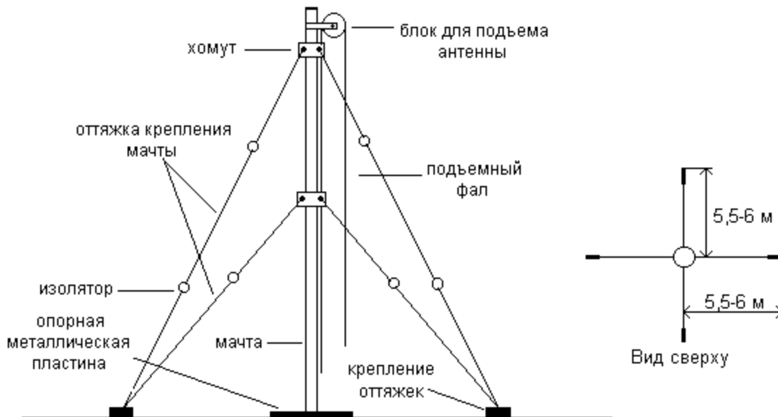
Рис. 2.11. Антенная мачта в развернутом виде
